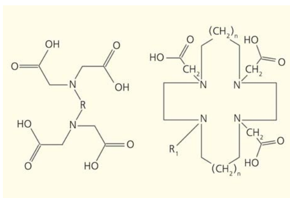
Рис.6. Ациклические и циклические комплексоны. Слева трилон Б R = (CH_2)_2 , справа DOTA ( n = 0 , R_1 = CH_2COOH ).
