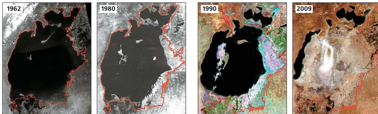
Сокращение площади Аральского моря.
