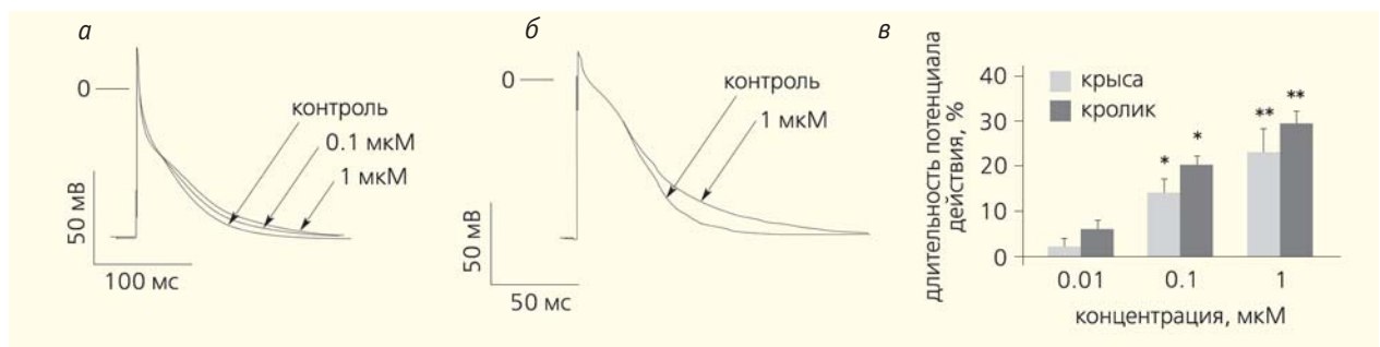
Рис.3. Записи потенциала действия предсердных кардиомиоцитов крысы (а) и кролика (б) при использовании ниферидила (в концентрациях 0.01, 0.1 и 1 мкмоль) и без (контроль). Видно, что ниферидил значительно дозозависимо увеличивал потенциала действия за счет замедления конечной фазы реполяризации в предсердных волокнах у каждого из животных, при этом в диапазоне исследованных концентраций ниферидил не изменял потенциала покоя и амплитуды потенциала действия. Такое увеличение длительности потенциала действия при неизменности других его параметров характерно для препаратов III класса и приводит к увеличению рефрактерности. На гистограмме (в) представлены средние данные по шести опытам для длительности потенциала действия на уровне 90% реполяризации, полученные на препаратах предсердий крысы (светлые столбики) и кролика.
