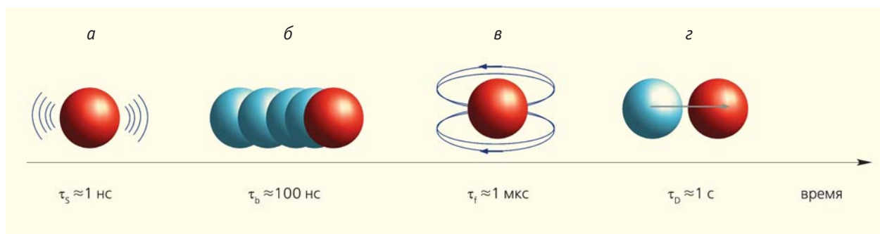
Рис.1. Иллюстрация процессов, происходящих при диффузии взвешенной частицы радиусом в 1 мкм в воде. Спустя наносекунду от произвольного времени начала отсчета формируется продольная звуковая волна, которая уносит около трети импульса частицы (а) [5, 6]. Около 100 нс частица продолжает двигаться, подчиняясь остатку импульса, которым она обладала в момент начала отсчета (б). Через приблизительно микросекунду формируется вязкий вихрь — поперечная волна возвращает частице часть отданного жидкости импульса; этот вихрь лежит в основе гидродинамической памяти (в). Спустя несколько секунд средний квадрат смещения частицы будет равен квадрату диаметра (г). Прекрасный обзор, посвященный динамике взвешенных частиц в растворе и роли гидродинамических эффектов, дан в [3].
