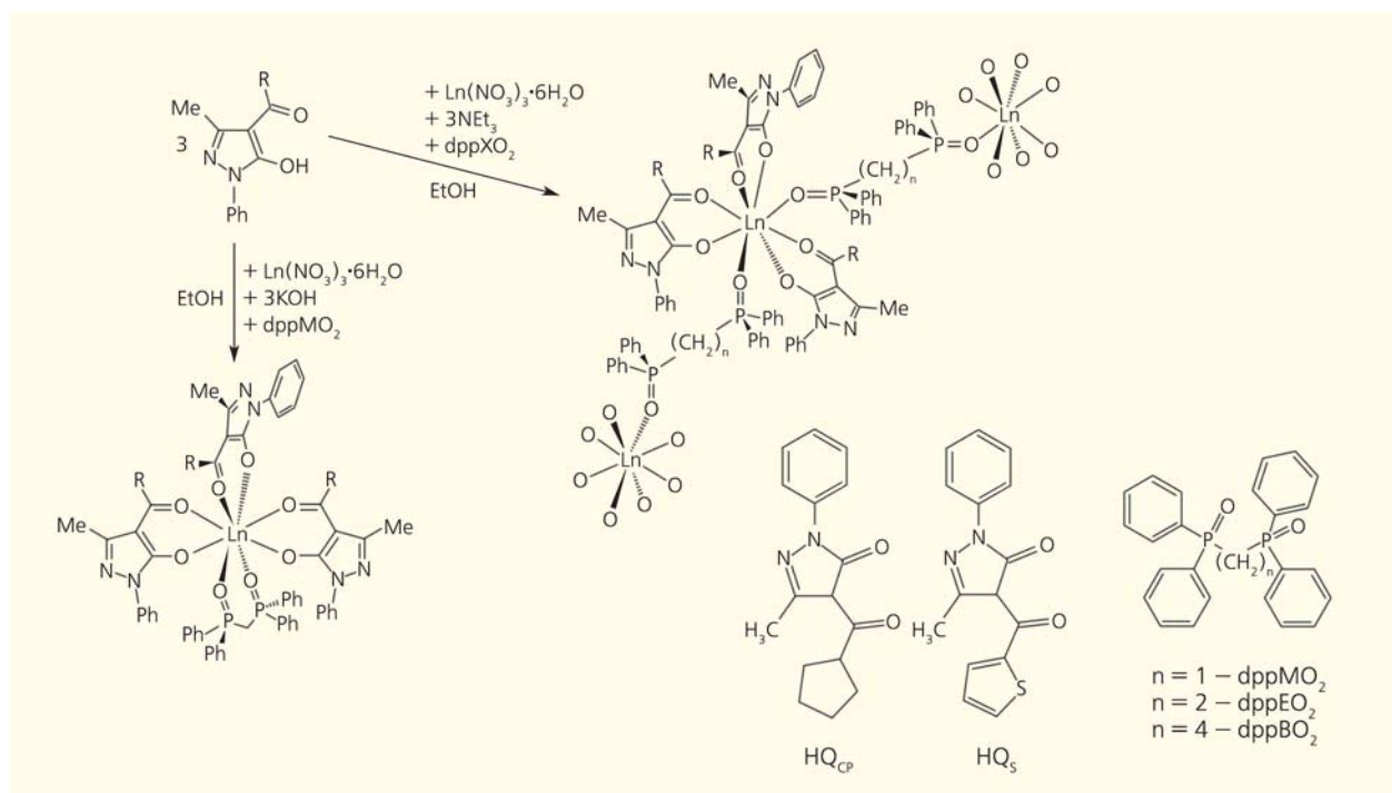
Рис.10. Моноядерные и полимерные ацилпиразолонаты редкоземельных элементов. Видно, что структура комплексов зависит от числа метиленовых звеньев (CH 2 ) в цепи мостикового лиганда dppXO 2 [8].
