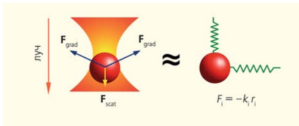
Рис.2. Броуновская частица, заключенная в лазерную ловушку. Луч лазера, падающий на частицу, благодаря отражению и преломлению порождает разнонаправленные силы. Под их действием частица ведет себя подобно гармоническому осциллятору и может быть описана законом Гука.
