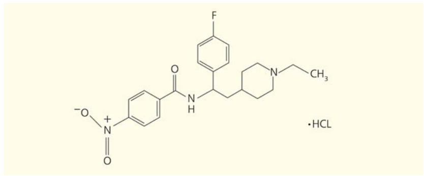
Рис.2. Структурная формула ниферидила [1].
