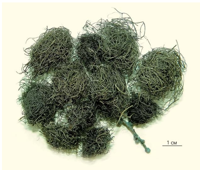
Эпифитные лишайники из зимних запасов красной полевки.
