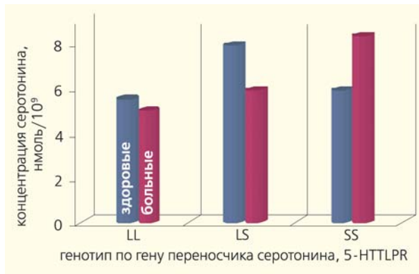
Рис.2. Вверху слева — зависимость концентрации серотонина в тромбоцитах от генотипа по гену переносчика серотонина (полиморфизм 5-HTTLPR, L — длинный аллель, S — короткий) у больных шизофренией и здоровых испытуемых; вверху справа — зависимость скорости связывания серотонина от генотипа по гену переносчика серотонина у больных и здоровых; внизу — зависимость концентрации серотонина в тромбоцитах от сочетания аллелей гена переносчика серотонина и гена MAOA (H — высокоактивный аллель, L — низкоактивный) у больных шизофренией.
