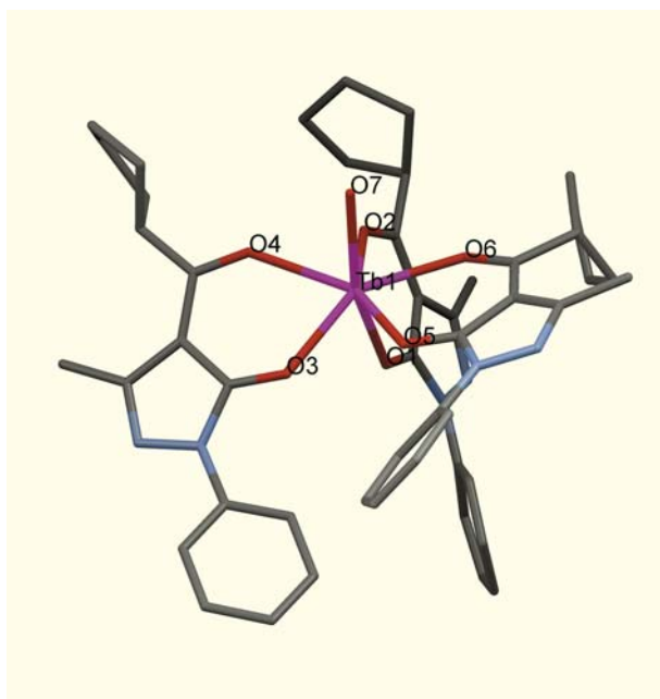
Рис.9. Кристаллическая структура гептакоординационного люминесцентного тербиевого комплекса Tb(Q_{CP})_3(H_2O) [7]. Атомы водорода скрыты для наглядности.
