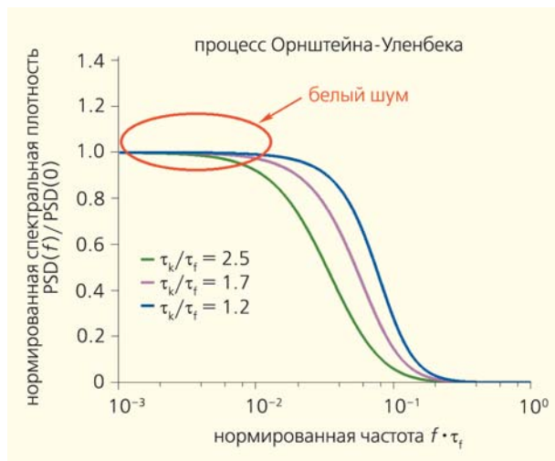
Рис.3. Спектральная плотность колебаний броуновской частицы в сильной лазерной ловушке, вычисленная в предположении верности теории диффузии Эйнштейна на сколь угодно коротких временных отрезках. Постоянство спектральной плотности на низких частотах соответствует случаю белого теплового шума.
