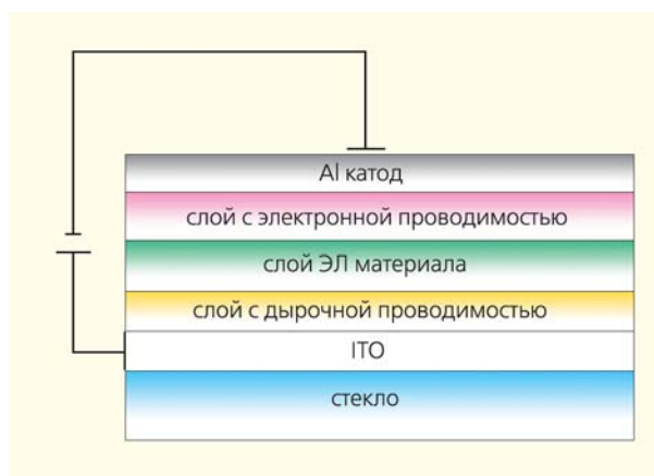
Рис.5. Многослойное OLED-устройство.
