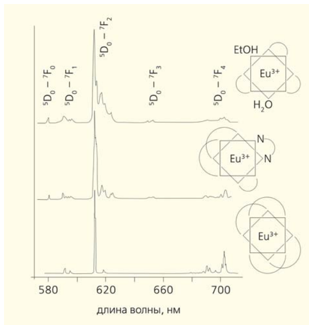
Рис.4. Люминесцентные спектры различных соединений \text{Eu}^{3+} с симметрией D_{4d} . Сверху вниз: \text{Eu}(\text{Qcp})_3(\text{H}_2\text{O})(\text{EtOH}) , \text{Eu}(\text{Qcp})_3(\text{phen}) , \text{NBu}_4[\text{Eu}(\text{Qcp})_4]^- . Справа схематично показано расположение лигандов вокруг центрального иона (полукруглыми линиями). Координирующие металл донорные атомы во всех случаях образуют квадратную антипризму [4].
