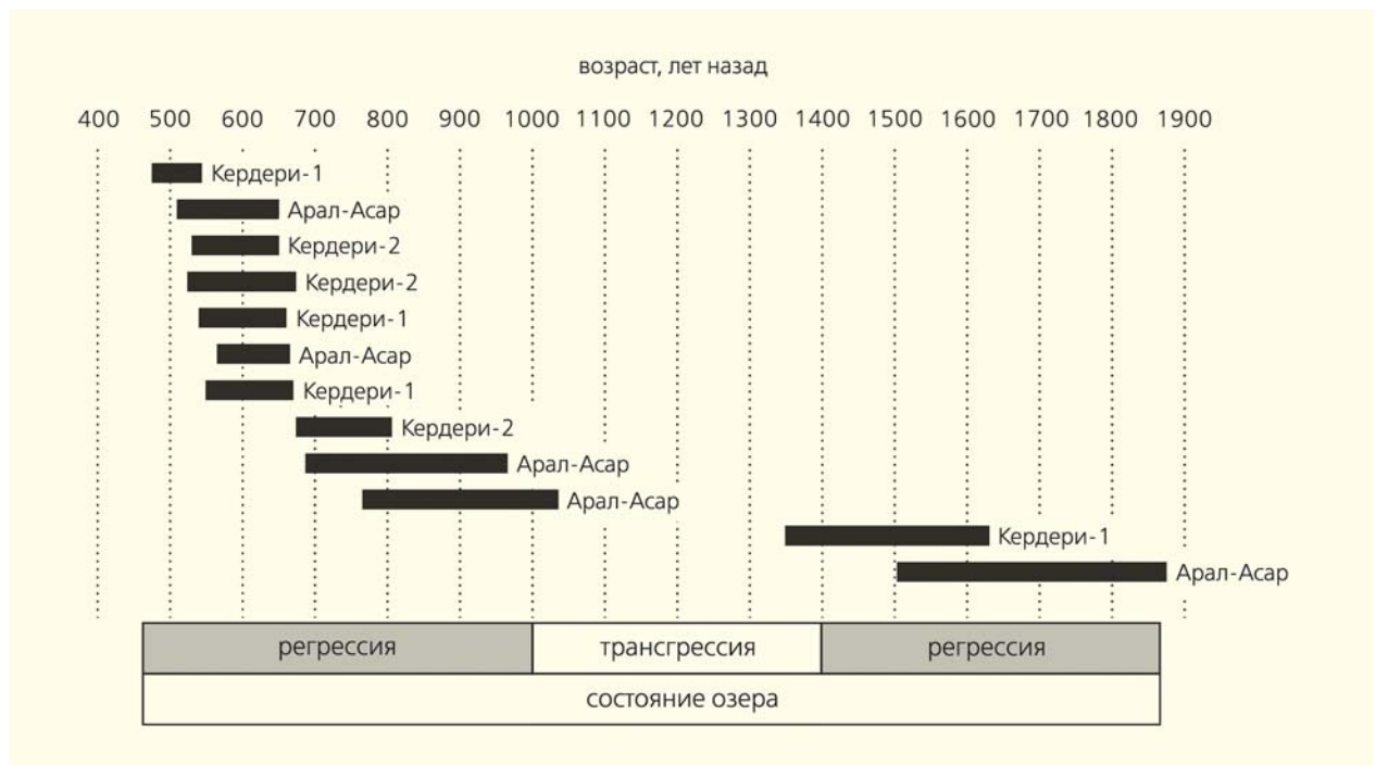
Результаты датирования находок из археологических памятников и реконструкция изменений уровня Аральского моря. Радиоуглеродные даты калиброваны и переведены в календарную шкалу времени.
