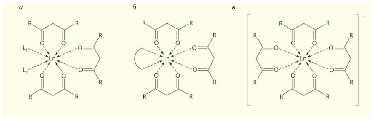
Рис.7. Строение обычных \beta -дикетонатных комплексов лантанидов: нейтральные комплексы с монодентатными (а) и бидентатными (б) дополнительными лигандами (обозначены полукруглой линией), комплексный анион (в).
