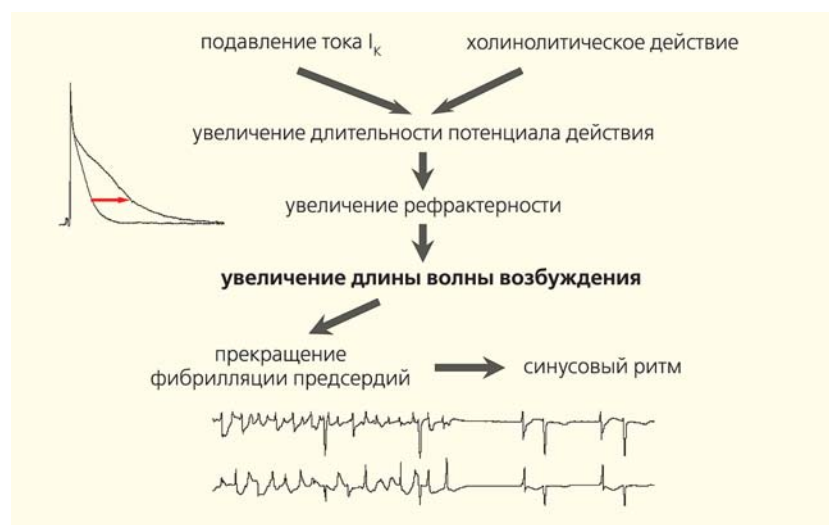
Рис.1. Механизм антиаритмического действия препаратов III класса.
