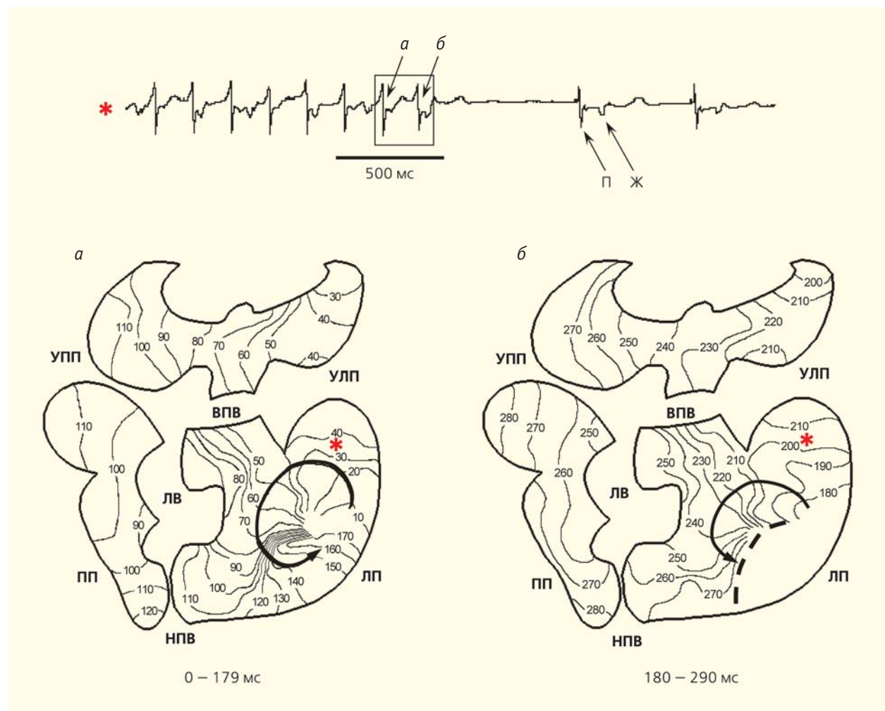
Рис.4. Результаты многоэлектродного электрического картирования предсердий, иллюстрирующие механизмы поддержания (а) и прекращения (б) мерцательной аритмии у собак под влиянием ниферидила (20 мкг/кг). На карте а видно, что мерцательная аритмия поддерживается благодаря циркуляции (ротации) возбуждения в свободной стенке предсердия вокруг некоторой границы раздела между зонами с большой и малой рефрактерностью. Все циклы мерцательной аритмии обусловлены подобным рода циркуляцией. Прекращение этого процесса (карта б) происходит в результате увеличения рефрактерности, благодаря чему «фронт» волны возбуждения встречает рефрактерный «хвост», ротация прекращается и восстанавливается нормальный (синусовый) ритм. П — активность предсердий; Ж — активность желудочков; а и б, включенные в квадрат, соответствуют картам тотального суправентрикулярного картирования (карты а и б). ВПВ и НПВ — верхняя и нижняя полые вены; УЛП и УПП — ушки левого и правого предсердия соответственно; ЛВ — легочные вены. Изохроны волн возбуждения на картах построены от 254 электродов с шагом 10 мс. Стрелками обозначена ротация волны возбуждения; пунктирной линией на карте б — область блокады распространения волны возбуждения в результате увеличения рефрактерности под действием ниферидила. Звездочкой на карте а обозначено место, где была зарегистрирована электрограмма, показанная вверху на вставке.
