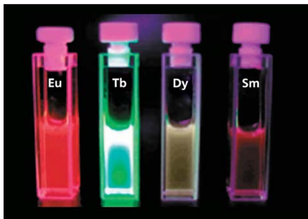
Рис.1. Растворы комплексов четырех лантанидов с наиболее выраженными люминесцентными свойствами — европия, тербия, диспрозия и самария в свете ультрафиолетовой лампы.
