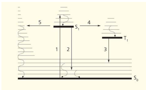
Рис.2. Схема квантовых переходов, обеспечивающих молекулярную люминесценцию. S_0 — основной электронный уровень (с колебательными подуровнями; показаны тонкими горизонтальными линиями), S_1 и T_1 — возбужденные синглетный и триплетный соответственно. Прямыми вертикальными стрелками обозначены поглощение (1) и излучательные переходы — флуоресценция (2) и фосфоресценция (3); горизонтальными стрелками — безызлучательные переходы: интеркомбинационное рассеяние (4) и внутренняя конверсия (5). Под действием кванта УФ-излучения молекула переходит из основного состояния S_0 в возбужденное синглетное состояние S_1 . Возврат из S_1 в S_0 соответствует флуоресценции. Излучение из более устойчивого во времени триплетного возбужденного состояния вызывает фосфоресценцию.
