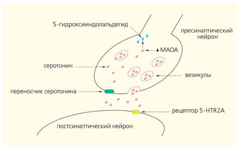
Рис.1. Транспорт серотонина в синапсе.
