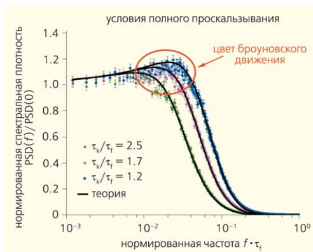
Рис.4. Спектральная плотность колебаний броуновской частицы в лазерных ловушках разной мощности, наблюдаемая в компьютерной модели. Чем ближе соотношение характерного времени ловушки \tau_k и характерного времени вязкого вихря \tau_v к единице, тем больше чувствительность к гидродинамическим явлениям. Для полноты рассмотрено два граничных условия между взвешенной частицей и жидкостью: условия полного проскальзывания, когда отсутствует обмен тангенциальной составляющей импульса на поверхности частицы между частицей и жидкостью (слева), и условия непроскальзывания жидкости (справа).
